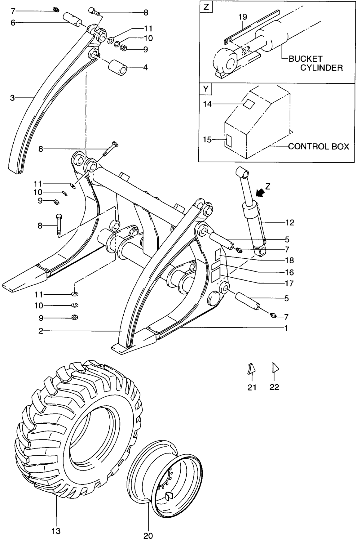
FIG. 158 LOGGER (TL047-648) 口カ -
