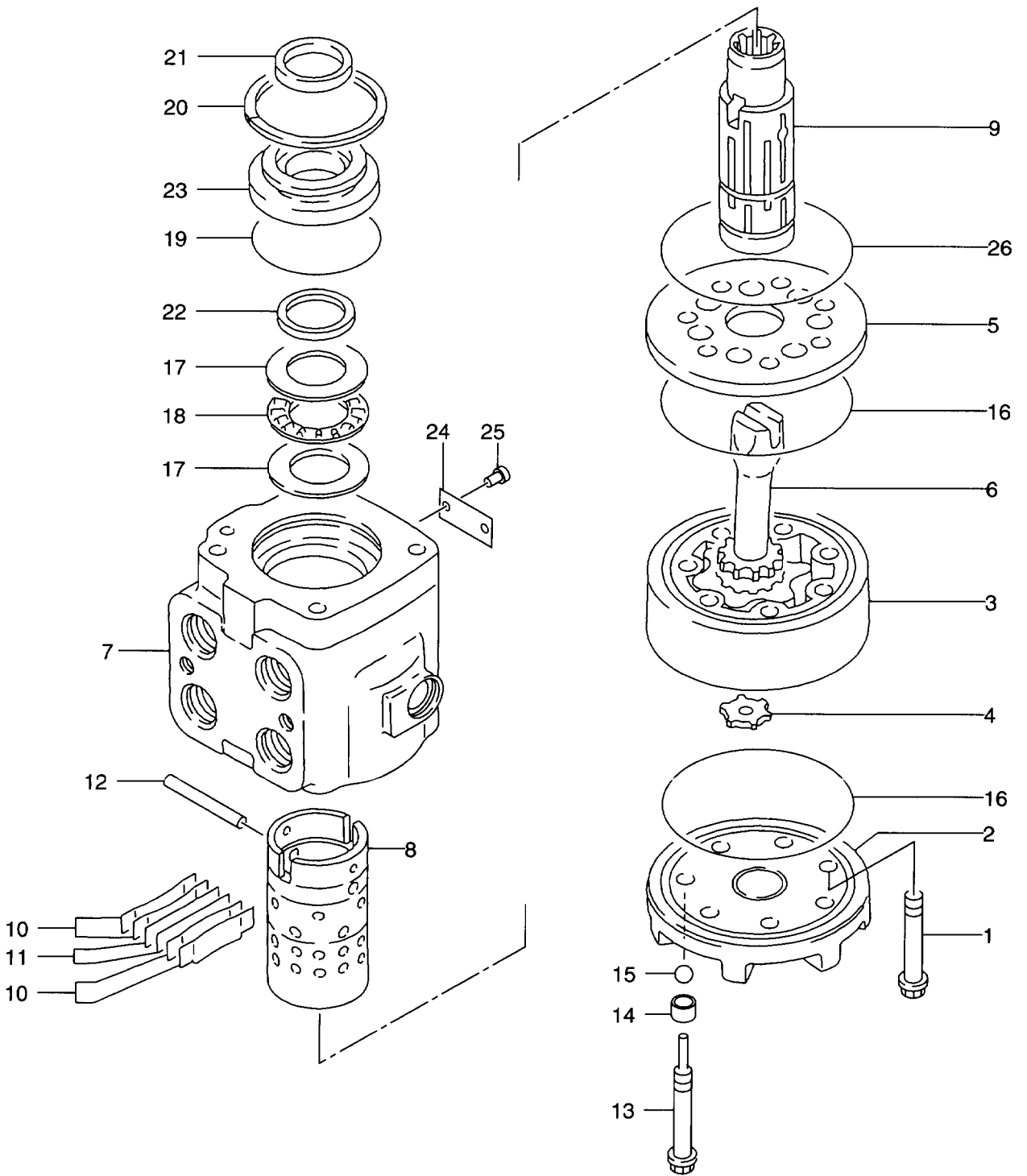
FIG. 65 STEERING VALVE (-2100) ステアリングバルブ
