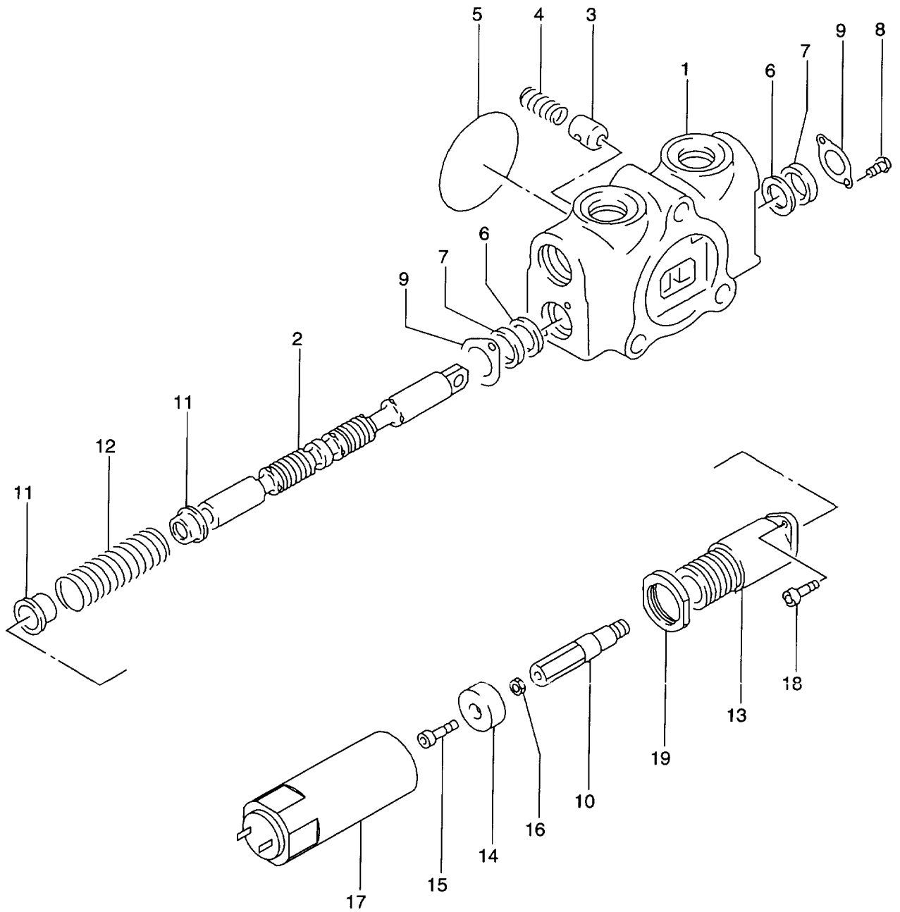
FIG. 119 CONTROL VALVE (BUCKET SECTION) (-1324) コントロールバルブ (バケツセクション)
