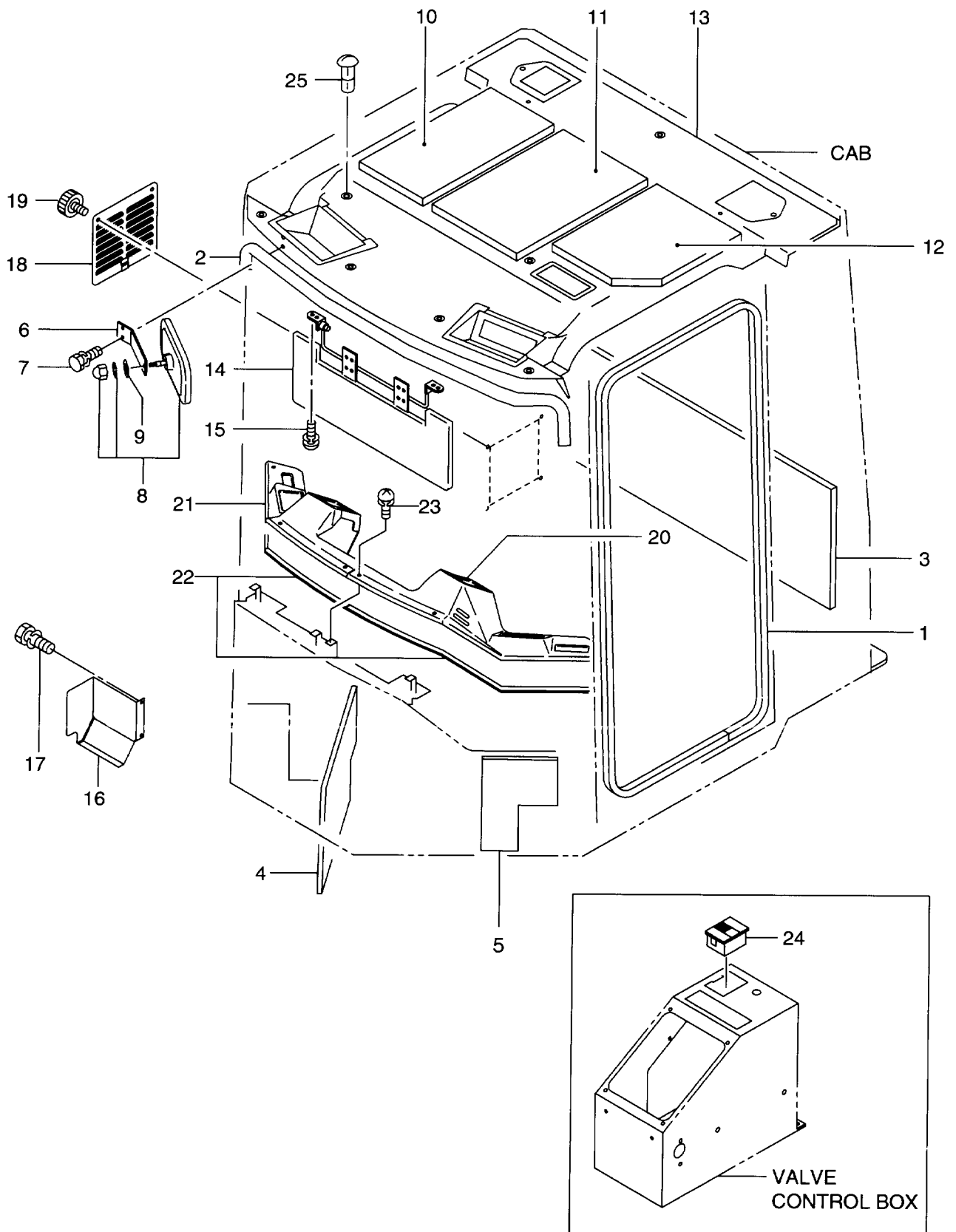
FIG. 96 CAB (COVER & MAT) (LCB150-648) (OP) キャブ (カバー&マット)
