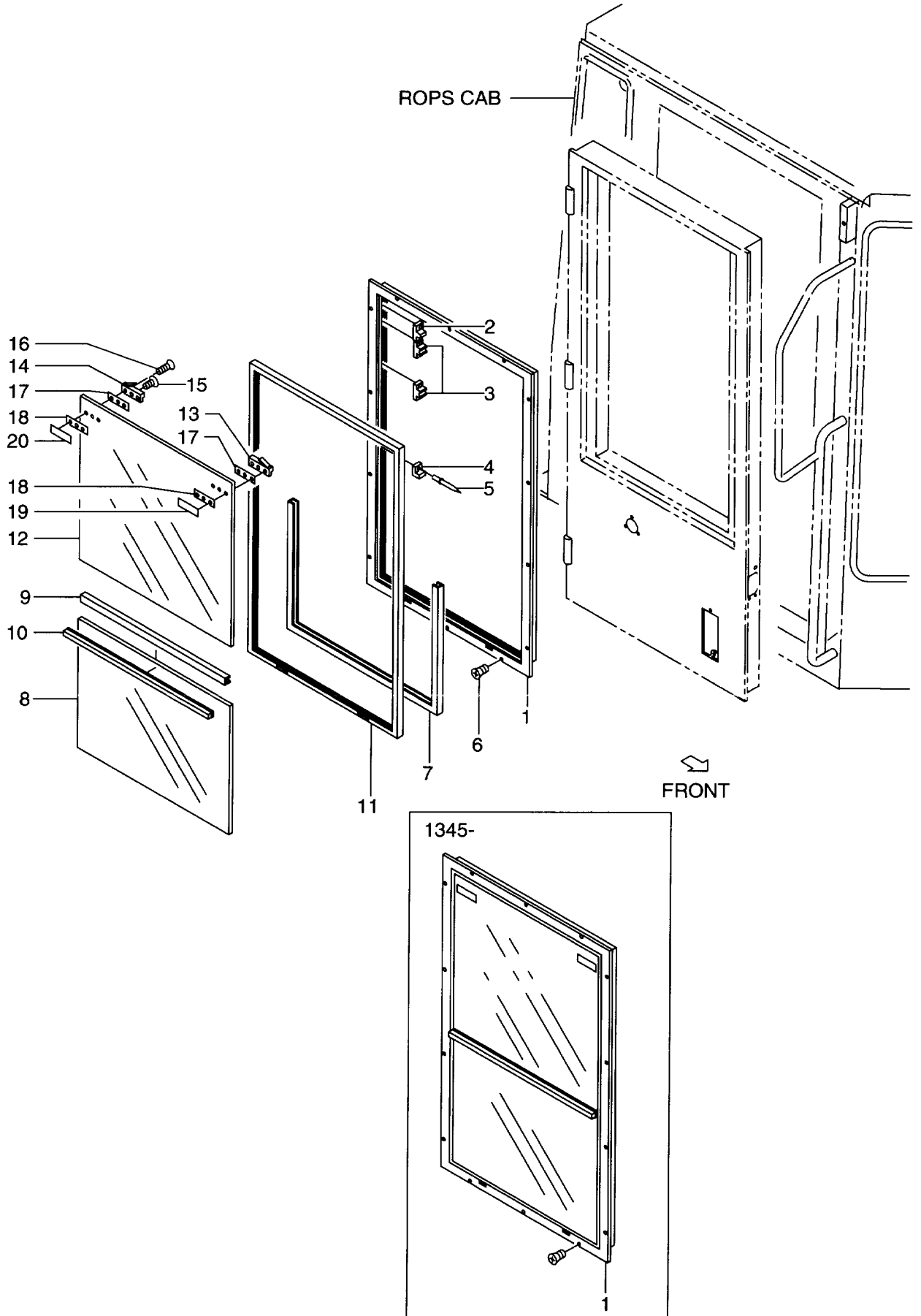
FIG. 77 ROPS CAB (DOOR,RH) (1/2) ロプスカブ(ドア)
