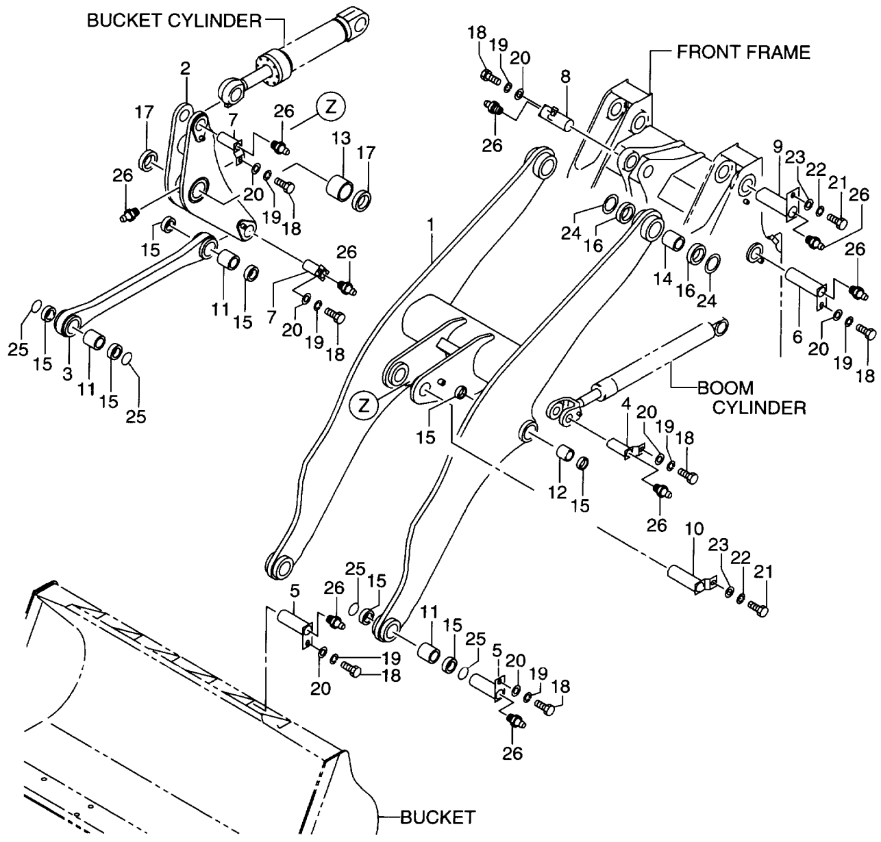
FIG. 137 BOOM ブーム
