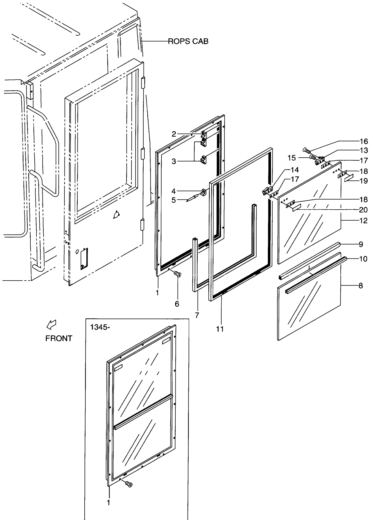
FIG. 79 ROPS CAB (DOOR,LH) (1/2) ROPSキャブ(ドア)
