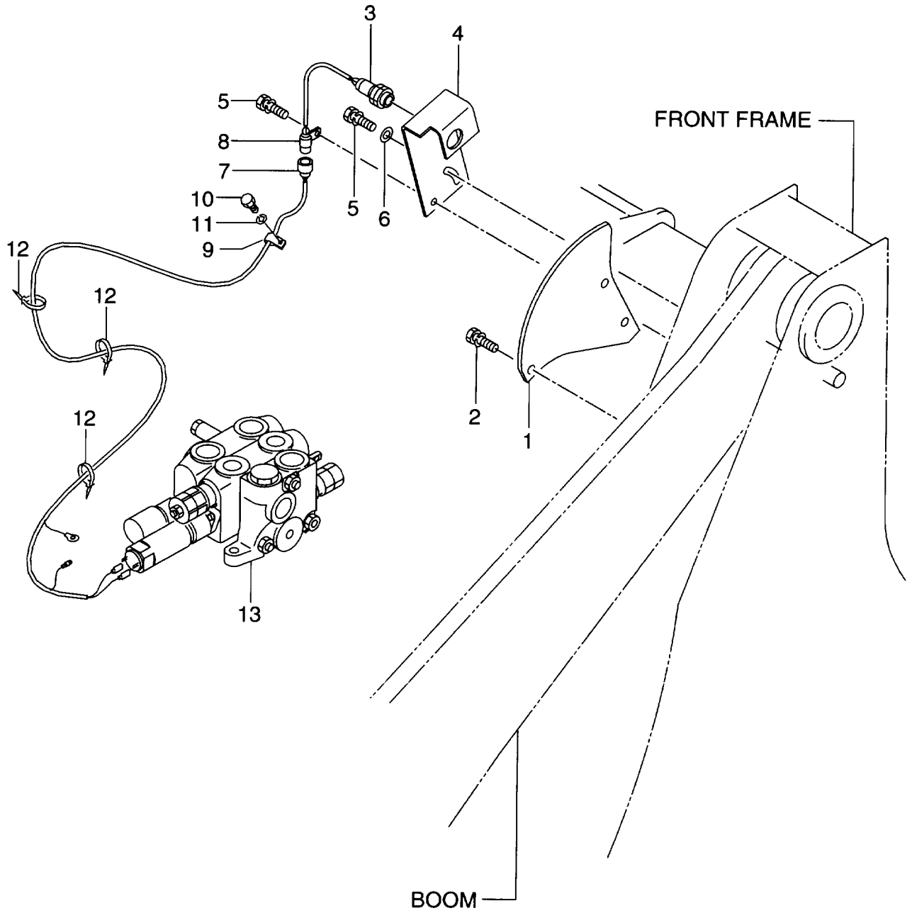
FIG. 139 BOOM KICKOUT ブームキックアウト
