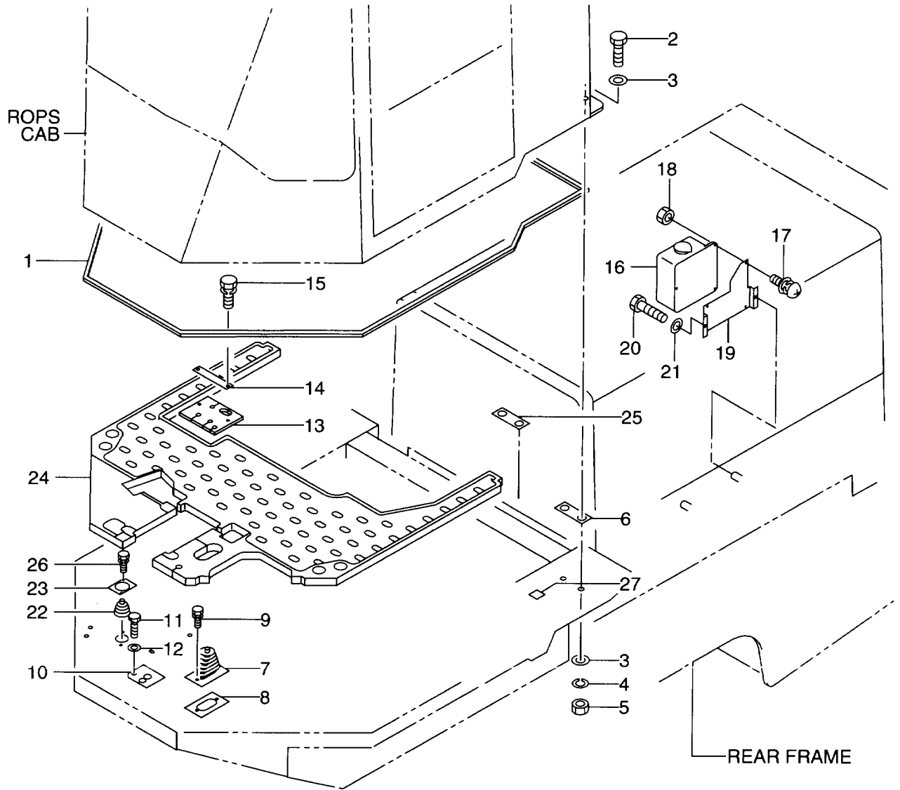
FIG. 84 ROPS CAB (MOUNT) ロブスカブ (マウント)
