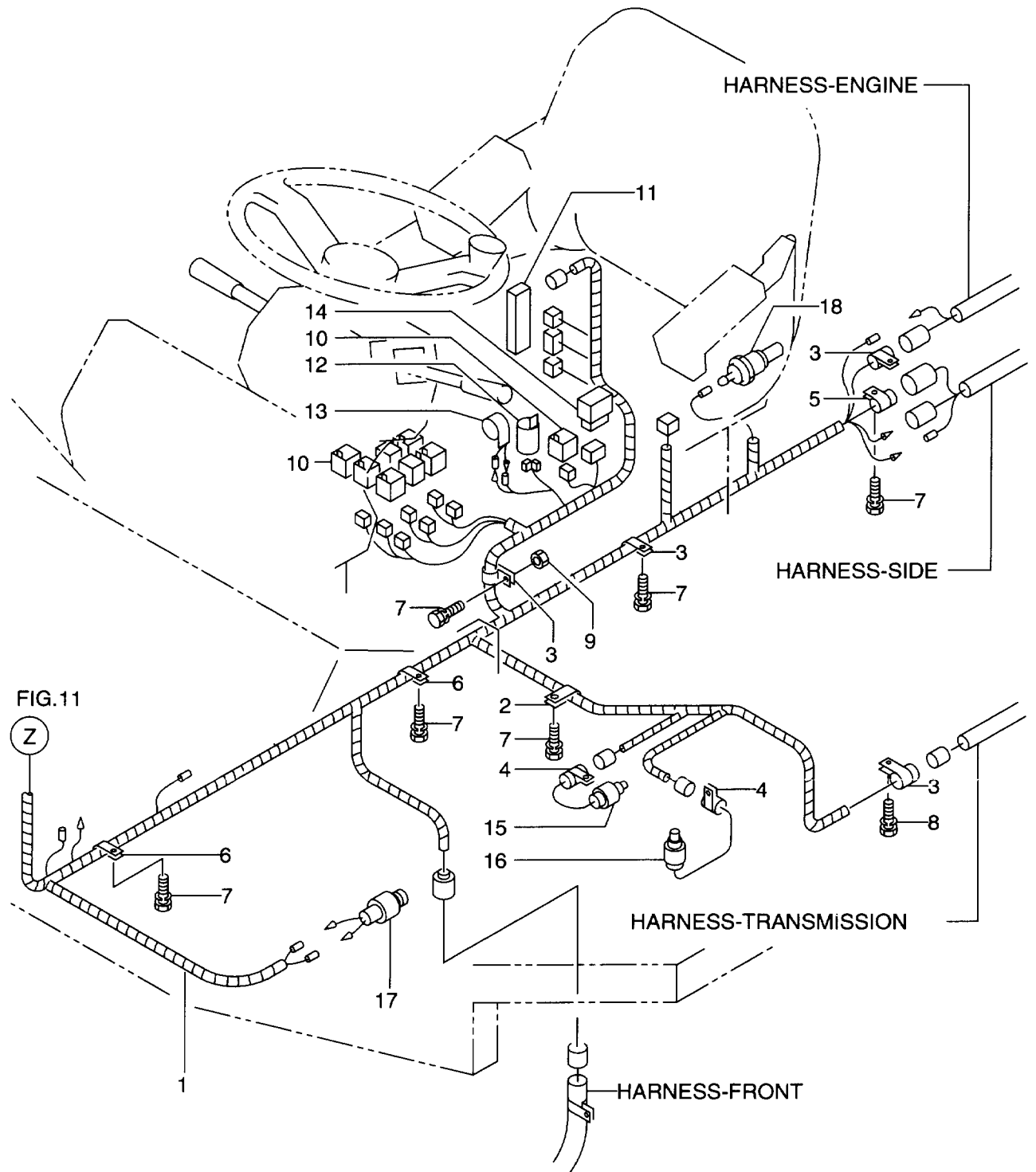
FIG. 10 WIRING (COCKPIT) (1/2) (-2100) ワイヤリング (コックピット)
