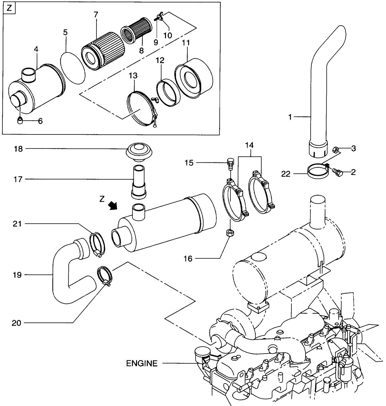
FIG. 7 AIR INTAKE & EXHAUST PARTS エア-インテーク&エキゾ-ストパ-ツ
