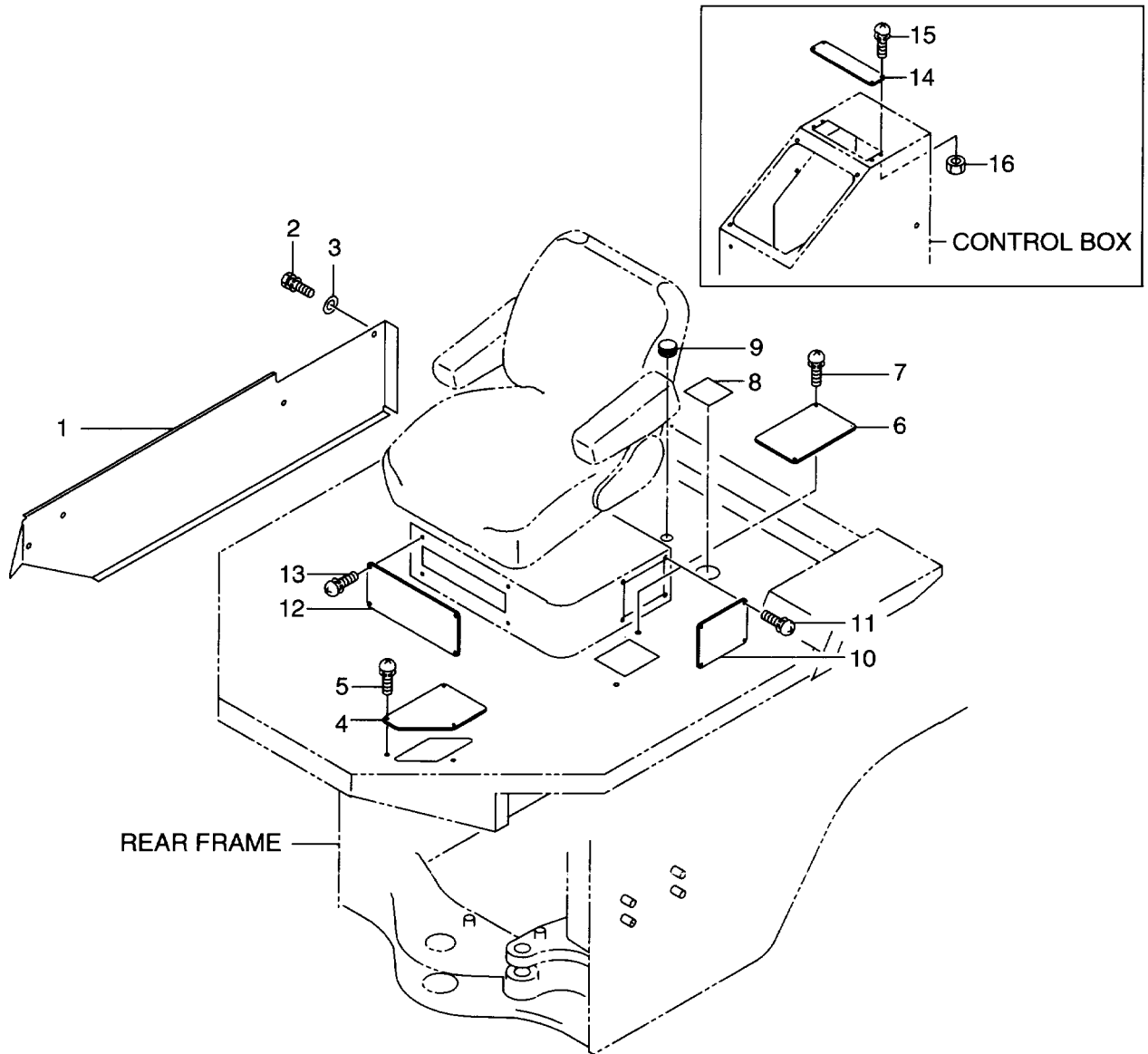
FIG. 112 AIR CONDITIONER LESS KIT(COVER)(ACLS3-648)(OP) エアコンディショナレスキット(カバー)
