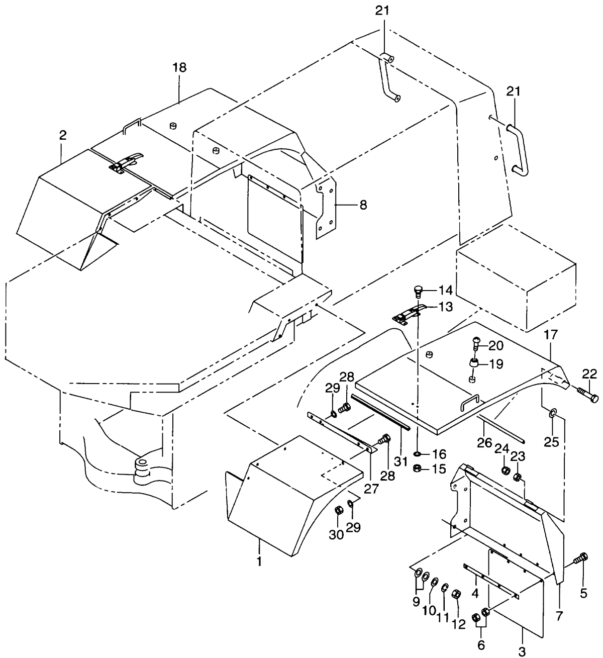
FIG. 114 FULL REAR FENDER (FRF-648) (OP) フルリヤーフエント
